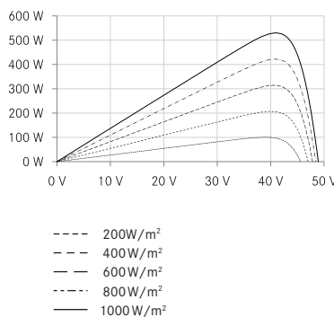
UP-diagram e.g. LX-525M/182-144+
