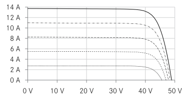
UL-diagram e.g. LX-525M/182-144+
